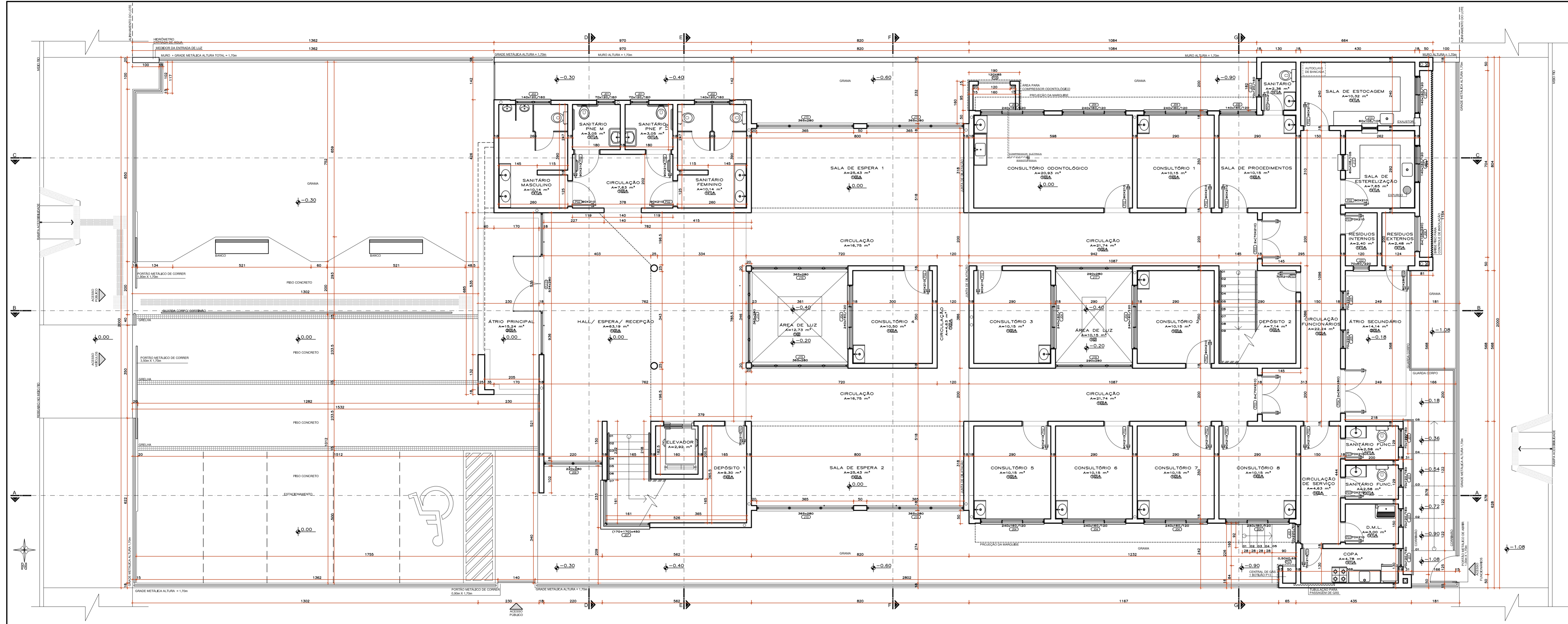
PLANTA BAIXA TÉRREO ESCALA: 1/75
