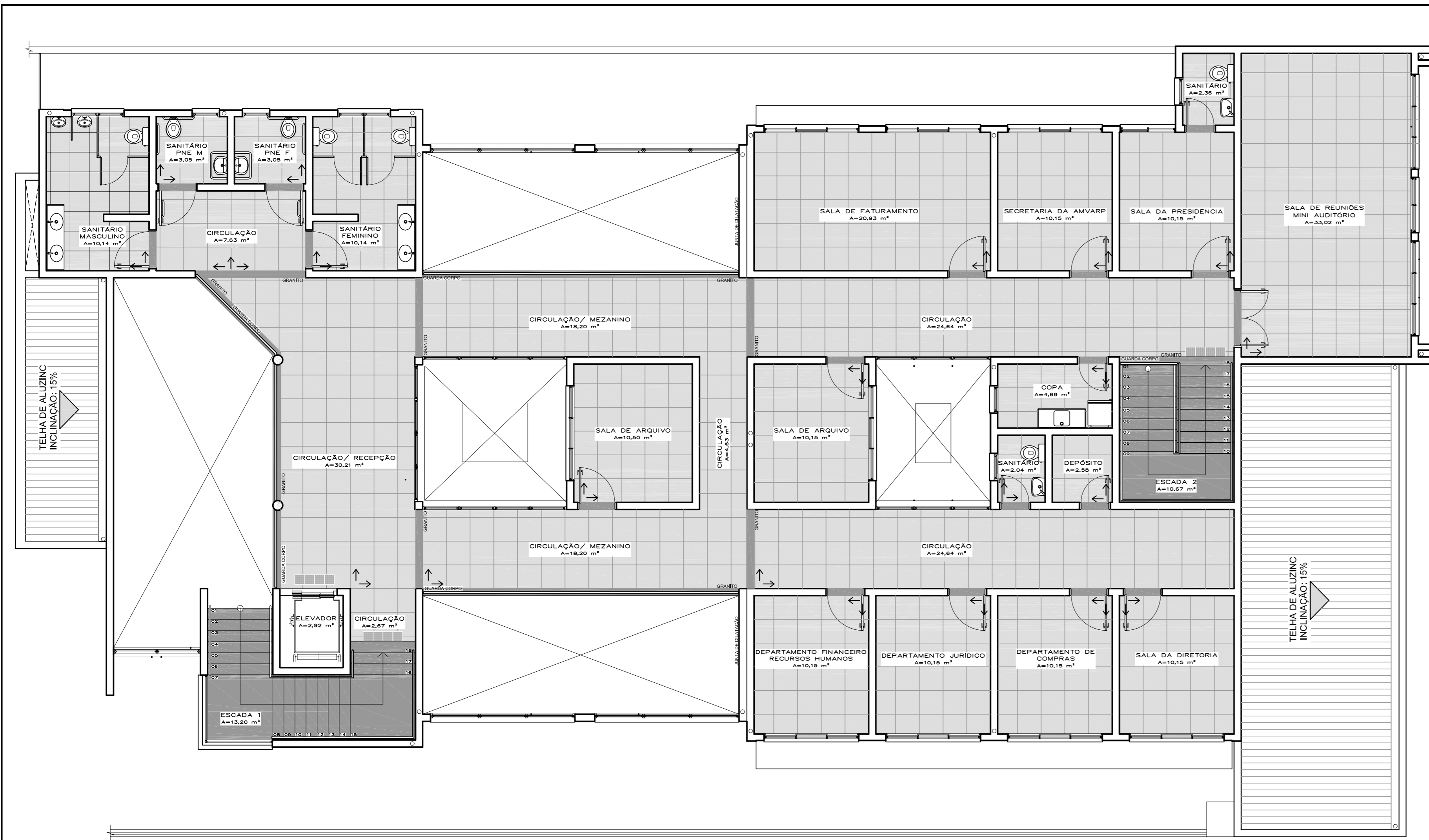
PLANTA BAIXA 2º PAVIMENTO ESCALA: 1:75
