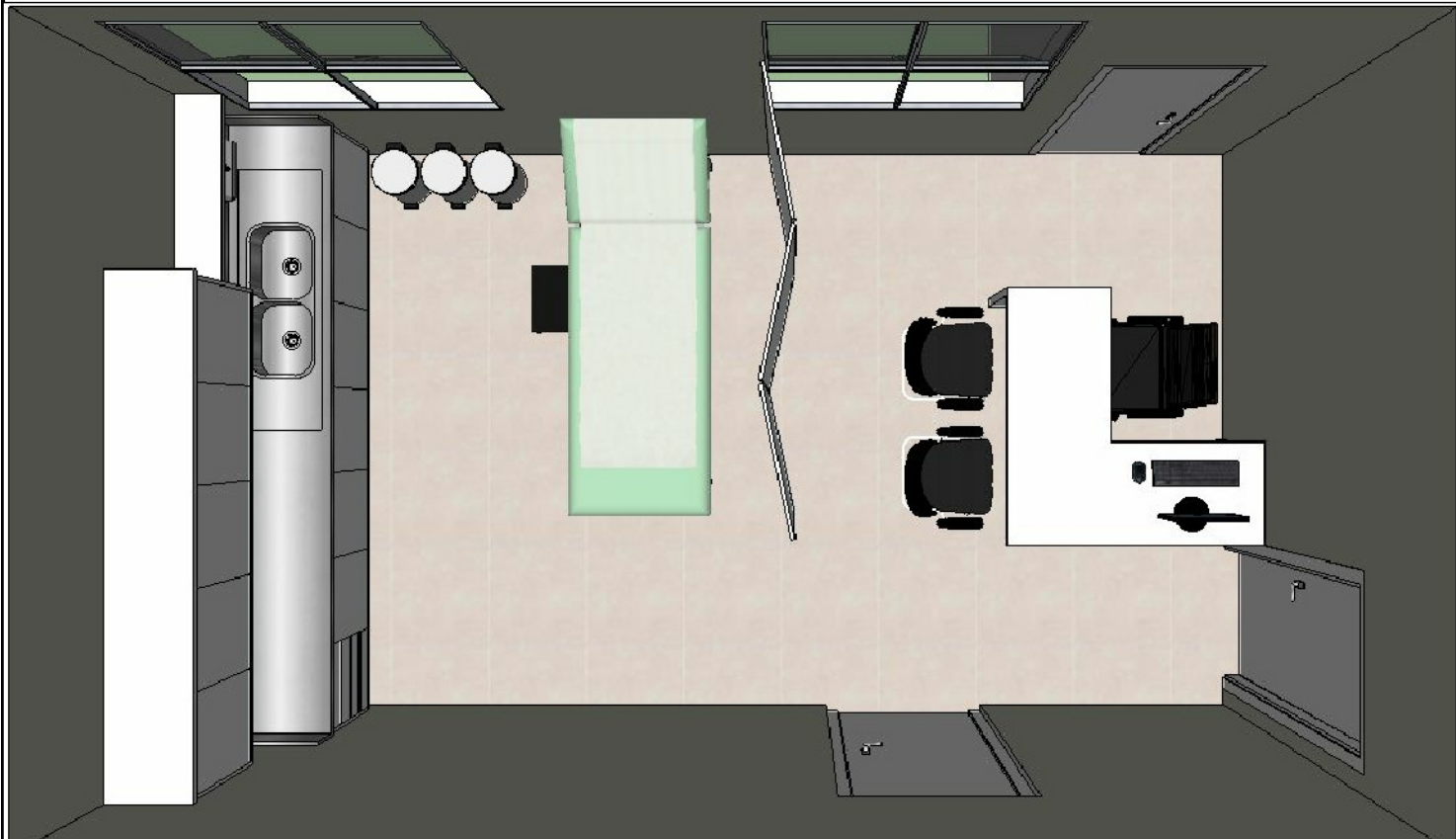
PLANTA BAIXA
