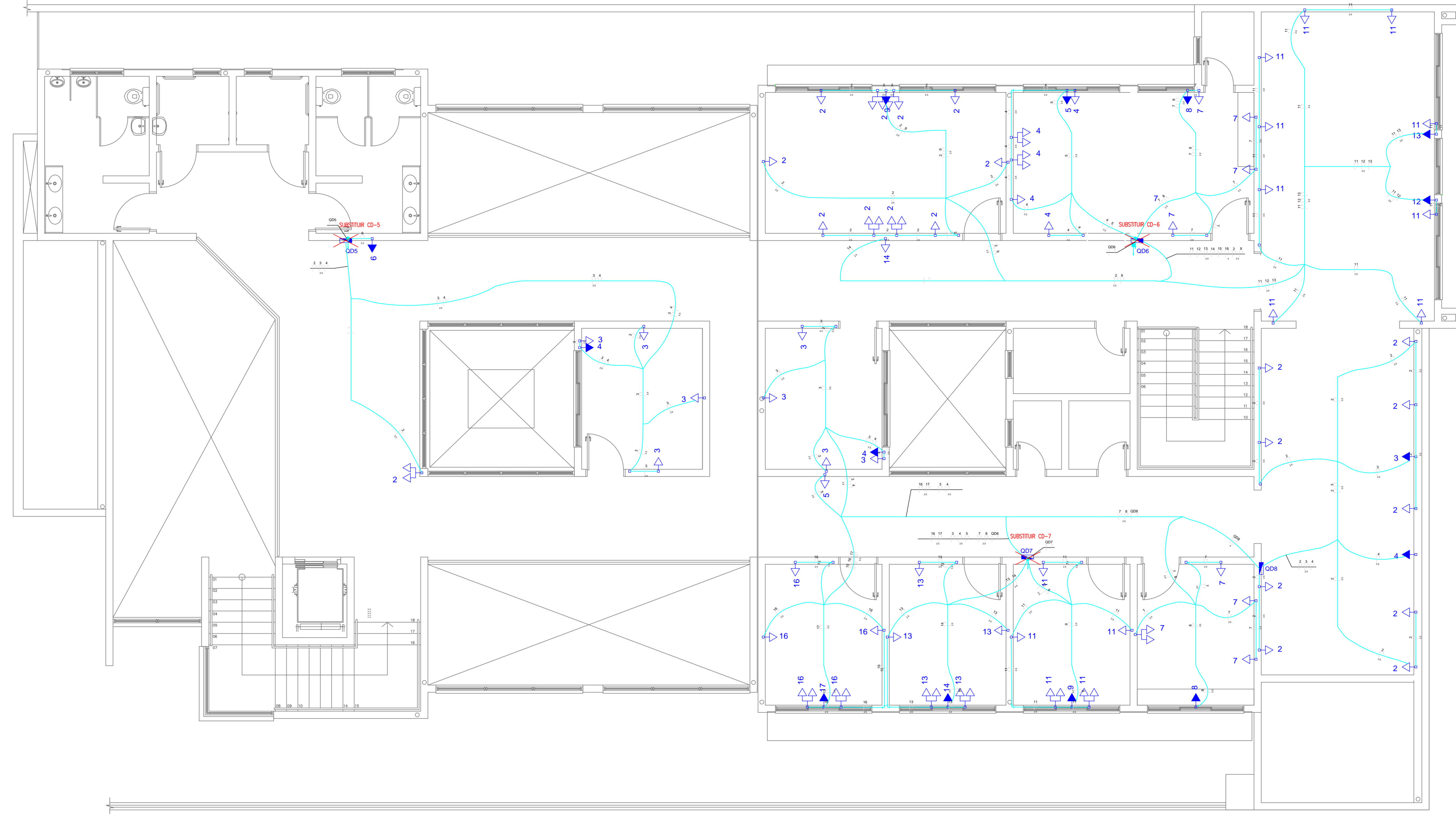
PLANTA BAIXA 2º PAVIMENTO ESCALA 1:50
