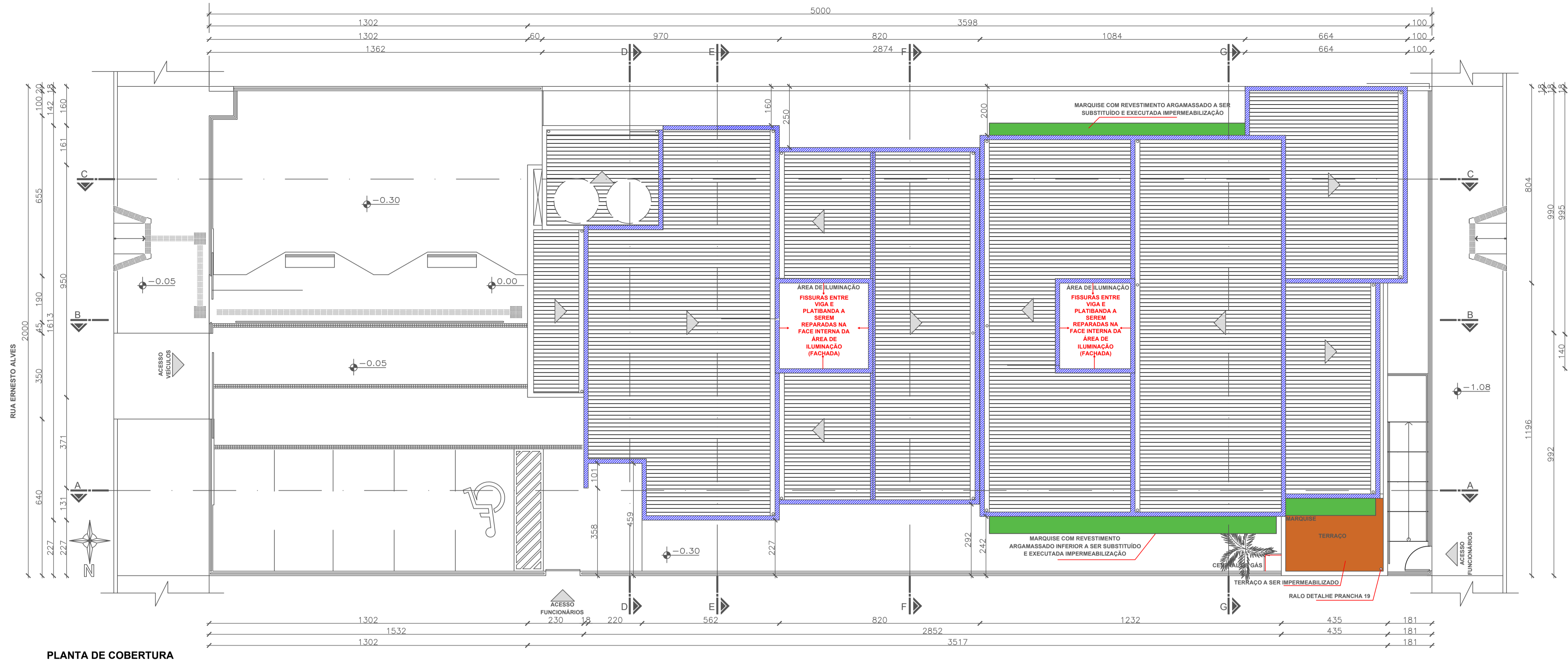
PLANTA DE COBERTURA
