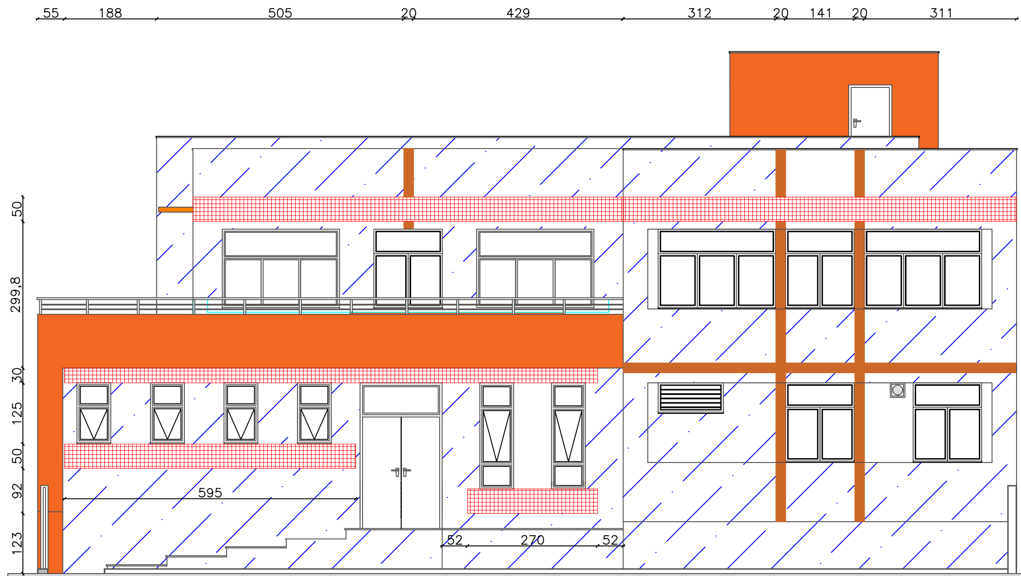
FACHADA OESTE - TRAV. VEREADOR WALTER KERN
