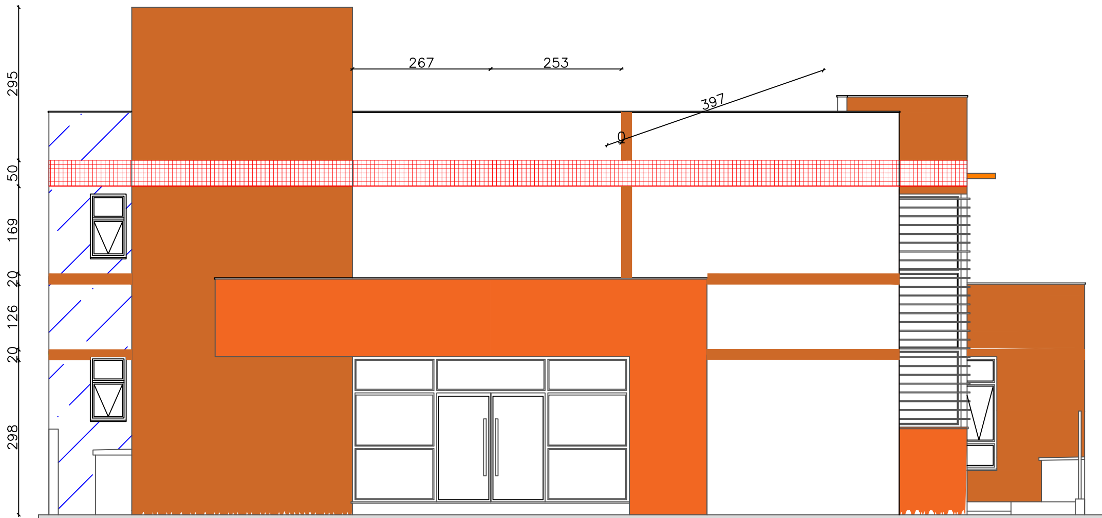
FACHADA LESTE - RUA ERNESTO ALVES
